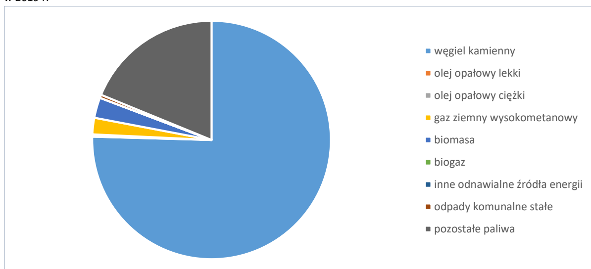
Wykres 16. Energia cieplna wyprodukowana przez przedsiębiorstwa ciepłownicze z podziałem według rodzajów paliw [GJ] w 2019 r.
