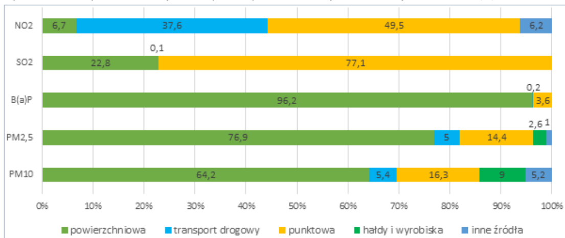
Wykres 19. Udziały źródeł w emisji zanieczyszczeń powietrza w województwie śląskim w 2019 r. (%)
